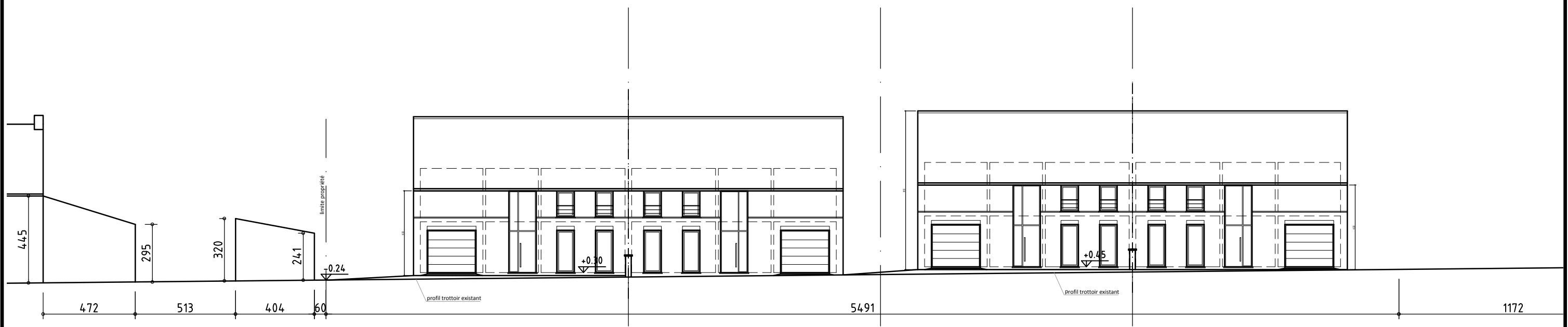
PROFIL RUE DES ECOLES Echelle 1/200
